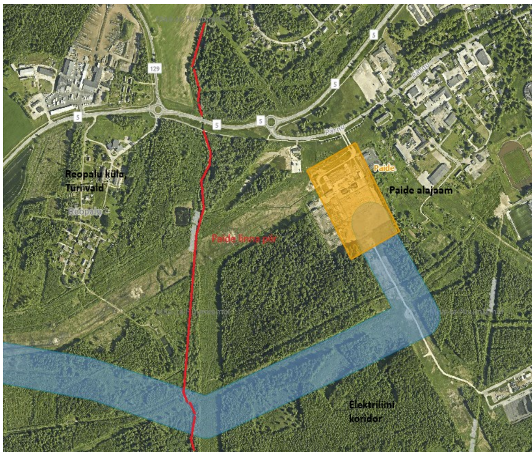
Skeem 1: Trassikoridor (sinisega) väljavõtte eriplaneeringu kaardirakendusest.
